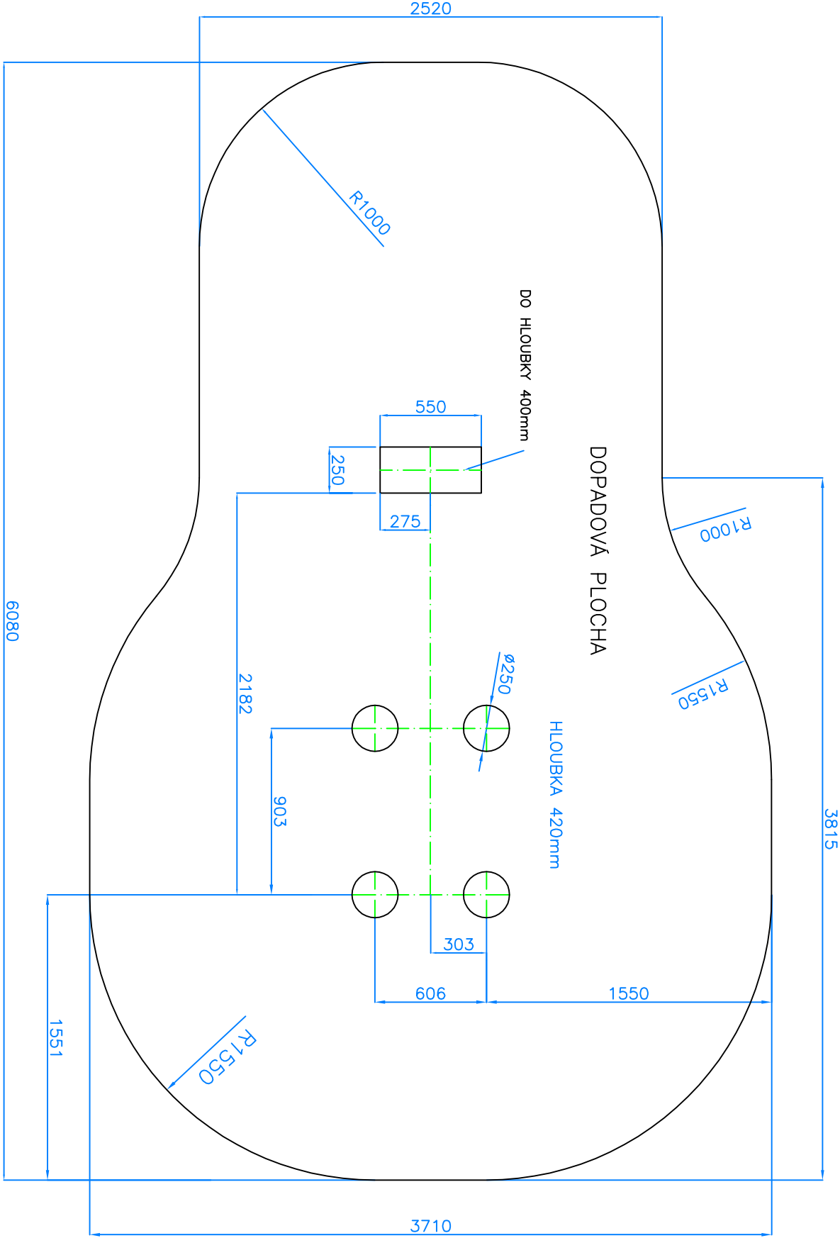
Príloha č.1. – Výkopové schéma včetně dopadové plochy
